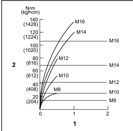
1. Festetid (sekunder) 2. Tiltrekingsmoment
