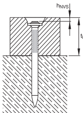
X-P_G3 MX, X-C_G3 MX: h_{NVS} = 2-3 \text{ mm}
